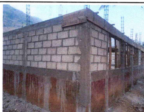
Foto 4: Vista parcial de la nueva estructura de concreto.
